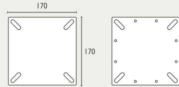
長穴タイプ
