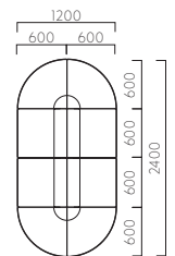
■上記施工例使用製品の寸法
