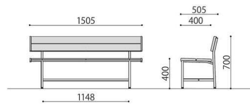
B-3(1500)
