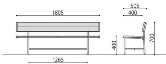
B-3(1800)
