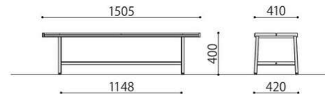
B-4(1500)
