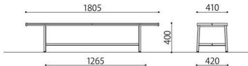
B-4(1800)
