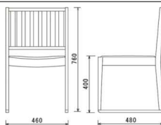
椅子 (W460・D480・SH400・H760)
