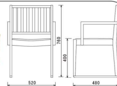
肘付椅子 (W520・D480・SH400・H760)
