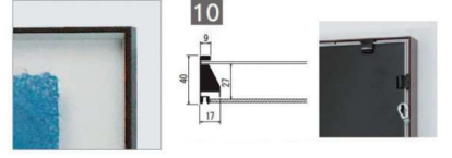
パネル(10)
