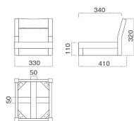
2268 小町 B カウンター椅子 (座厚 110mm) 張地：クレنزⅡ L-6682 (A)
