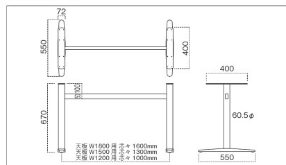
天板適用サイズ D600～D750 用
