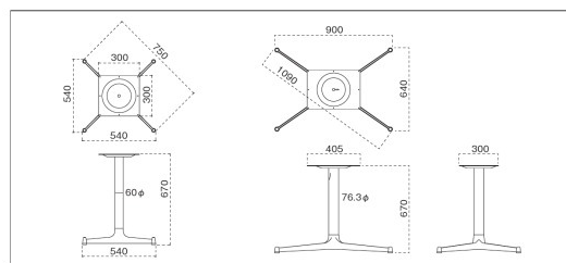
天板適用サイズ D700～D750 用
