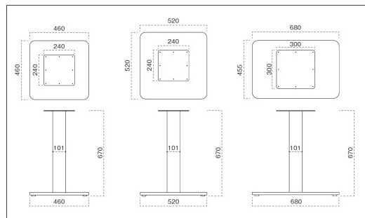
天板適用サイズ D600～D900 用
