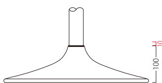
脚部:GT-850~851 ポール:38φ
