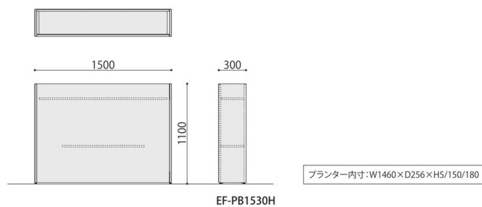
EF-PB1530H
