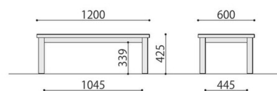
EF-OT1260
