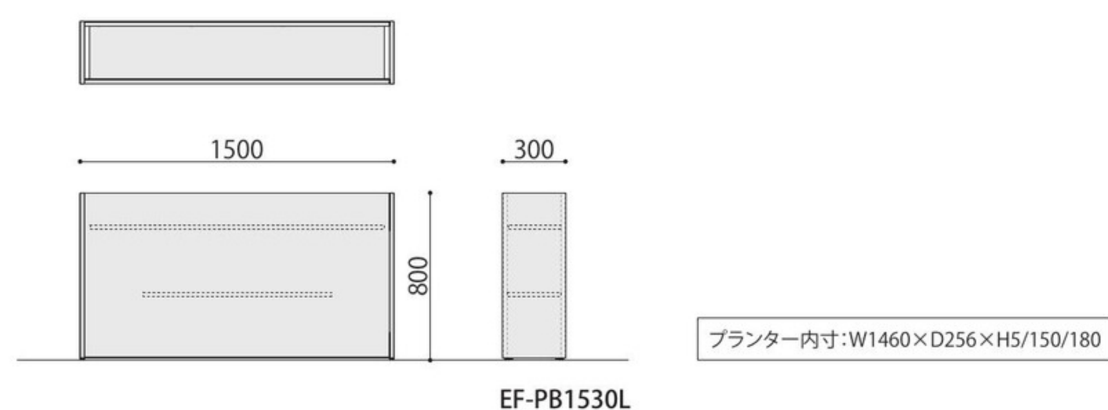
EF-PB1530L
