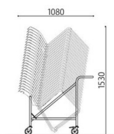
MK-480 (12台) 積載時
