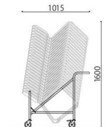
SFIDA (12台) 積載時
